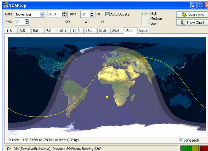
Fig.1 Long path centrato con OM3PA riferito al caso 1, tracciato con il programma VOAProp di G4ILO http://www.g4ilo.com/voaprop.html
