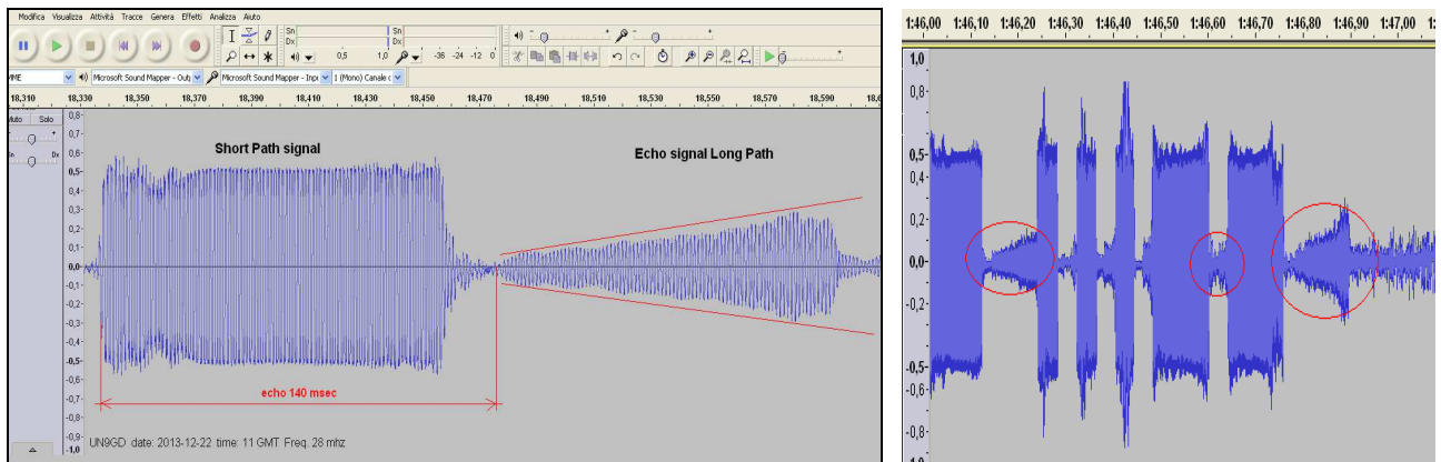
Fig.17. Caso 5. Ricezione da parte di IK2GRA del segnale di UN9GD dal Kazachistan, dove si vede l'andamento conico dell'ampiezza del segnale eco, ritardato di 140 msec. rispetto al segnale (linea CW) che l'ha generato. L'ampiezza del segnale eco, in questo caso aumenta di un fattore 3. La traccia audio, della durata di circa 2 minuti e mezzo, presenta quasi sempre un andamento crescente dell'ampiezza del segnale eco, come evidenziato nell'immagine a destra dove si vede un estratto piu' lungo del tracciato audio. Credits:IK2GRA
