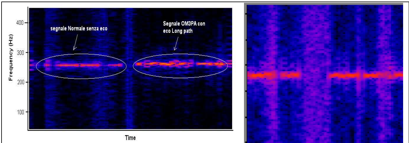
Fig.15. Analisi del segnale di OM3PA che evidenzia un minidoppler ionosferico con allargamento della traccia. L'immagine a destra mostra un ingrandimento della traccia CW. Analisi effettuata con WINRAD.
