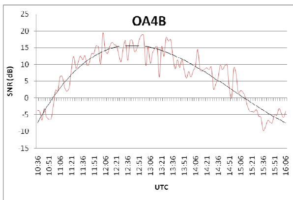
Fig.19 Grafico dell'andamento del segnale dei due beacons monitorati. OA4B è sempre stato ascoltato via Long path, mentre il beacons ZL6B È stato ascoltato sempre via Short Path (eccetto alcuni passaggi Long path di breve durata). La curva nera rappresenta una linea polinomiale che evidenzia un andamento gaussiano del segnale.
