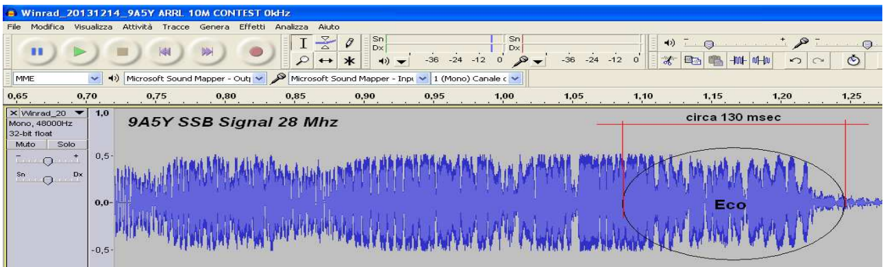
Fig 10. Analisi di una porzione di segnale di 9A5Y in 28 mhz SSB registrato durante l'ARRL 10 Metri contest 2013. Il segnale era riconoscibile in quanto presentava un forte eco. (9A5Y data ricezione 14.12.2013 ore 12.21 UTC). Credits: IK3XTV
