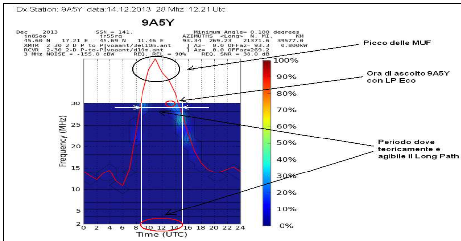
Fig.12. Esempio di analisi del percorso e delle MUF effettuato sempre con VOACAP e riferito all'ascolto di 9A5Y. (MUF Voacap vedi note 3)
