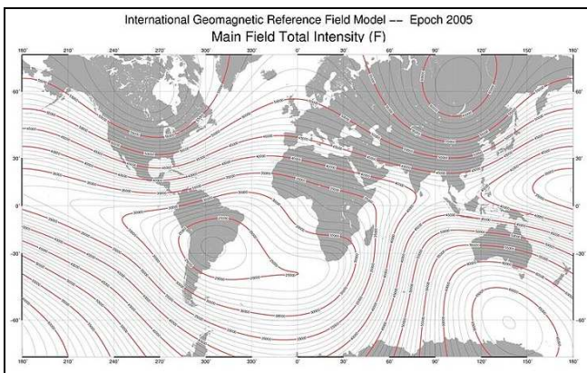
Fig.16. Il campo magnetico terrestre non è uniforme e presenta delle significative variazioni sia in intensità che direzione. Inoltre sono documentate anche significative anomalie crostali. Credits: Wikipedia http://it.wikipedia.org/wiki/File:F_map_mf_2005_large.jpeg
