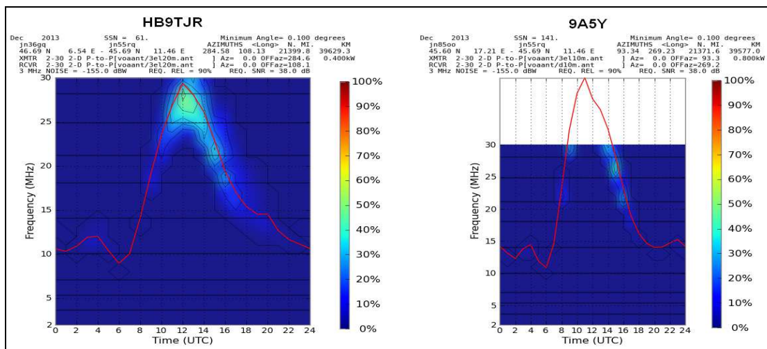
Fig.14. Analisi delle MUF e della fattibilità teorica del collegamento long path con il programma VOACAP di HB9TJR e di 9A5Y, con il software di previsione che conferma gli orari long path ed evidenzia l'apertura del percorso LP in prossimità del picco massimo delle MUF (3), che raggiungono il picco proprio attorno agli orari della registrazione degli echi (curva Rossa)
