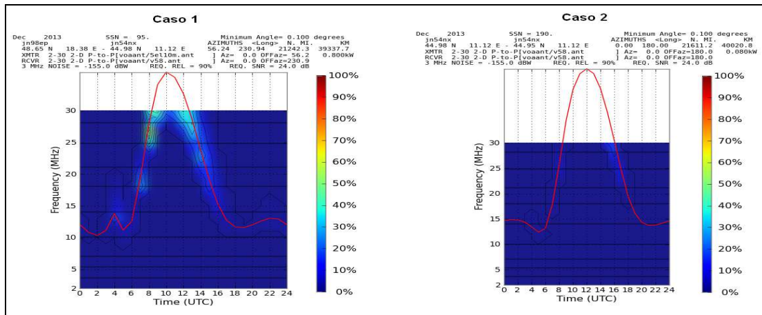
Fig.13. Analisi delle MUF e della fattibilità teorica del collegamento long path con il programma VOACAP. Sono stati analizzati il caso 1 e il caso 2. Con il software di previsione che conferma gli orari long path ed evidenzia l'apertura del percorso LP in prossimità del picco massimo delle MUF (3), che salgono proprio attorno agli orari della registrazione degli echi (curva Rossa).
