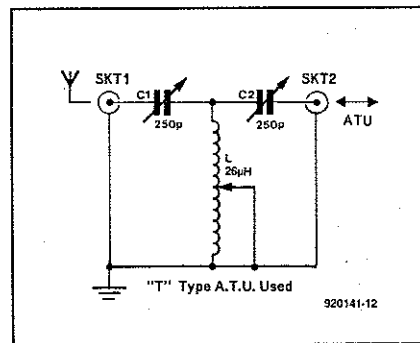
Fig. 2. Type 'T' ATU used.
